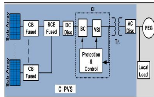
Fig. 5 CI PVS
