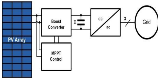
Fig. 3 DC-PV PVS
