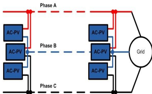
Fig. 4 AC-PV PVS
