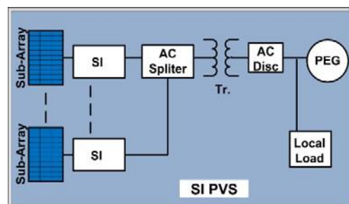
Fig. 6 SI PVS
