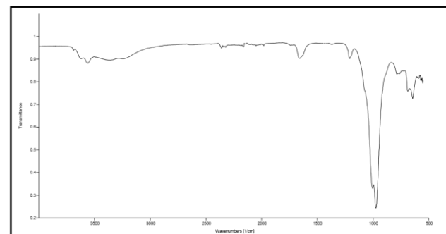
Fig. 6 Sepiolite
