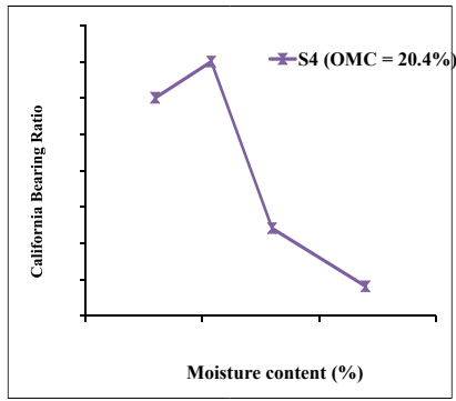
Fig. 2 (d) The CBR versus the moisture content for soil sample S4
