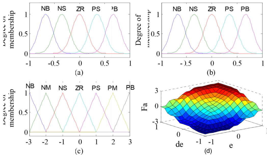
Fig. 3 MFs for FLC (a) Input side, ; (b) Input side, ; (c) Output side, F ; (d) Surface plot
