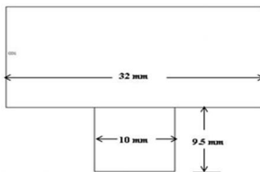
Fig. 3 Pin dimensions
